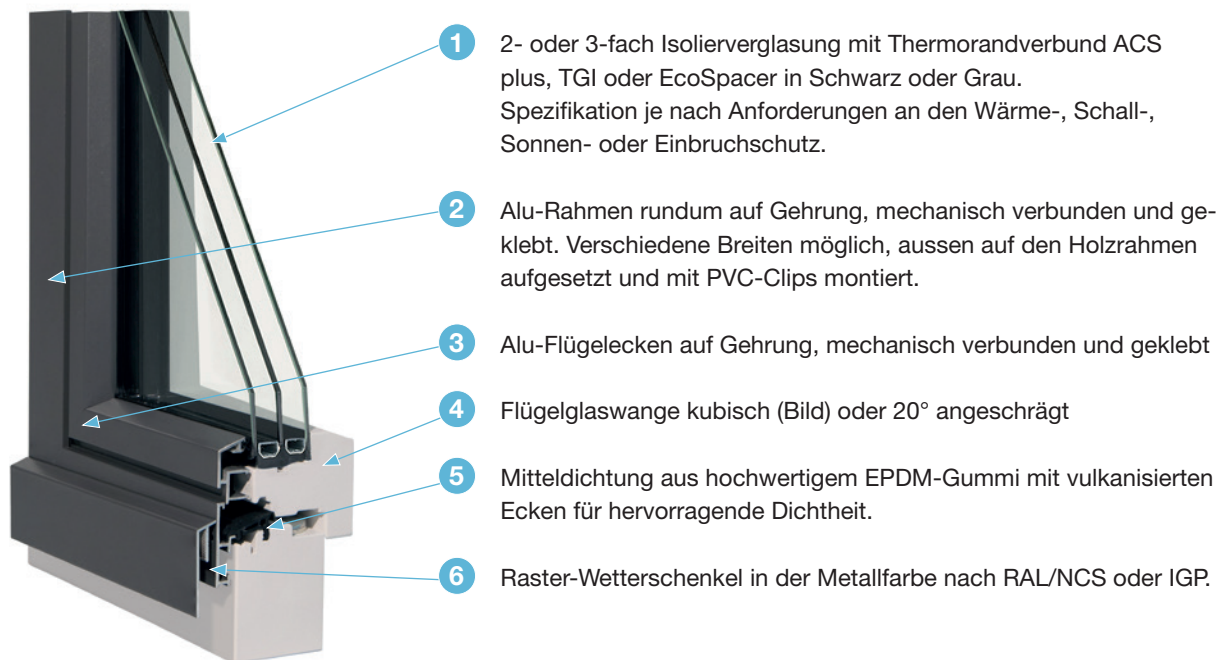
Metallflügelprofile Standard-schräg und flächenbündig
